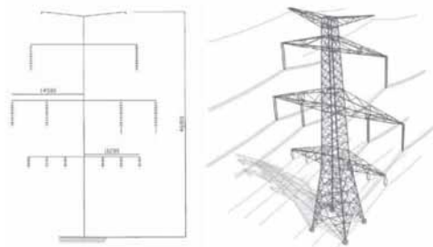
Sloučené vedení 2 \times 400 kV a 2 \times 110 kV na jednom stožáru, preferovaná Varianta I.
